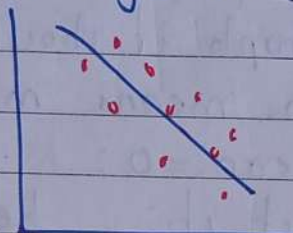
linear ✓
